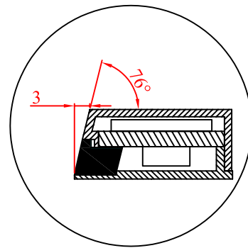
Detail A-A 6:1
