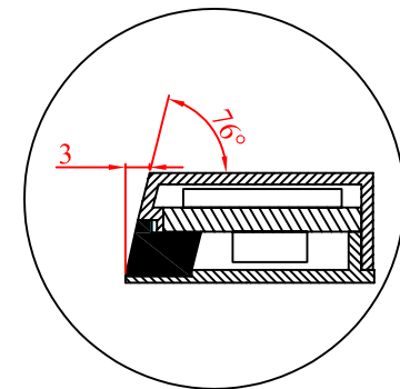
Detail A-A 6:1
